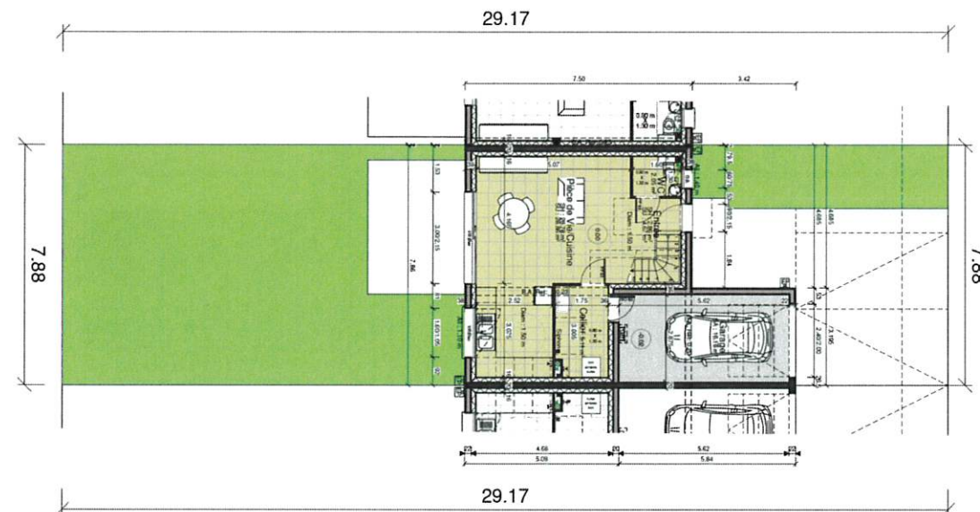
Plan de masse - sans échelle
