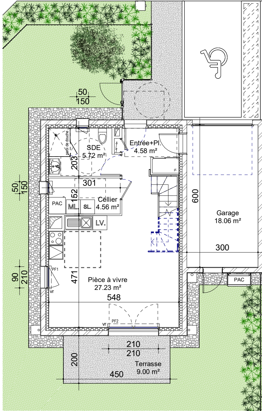
RDC - 1/100
