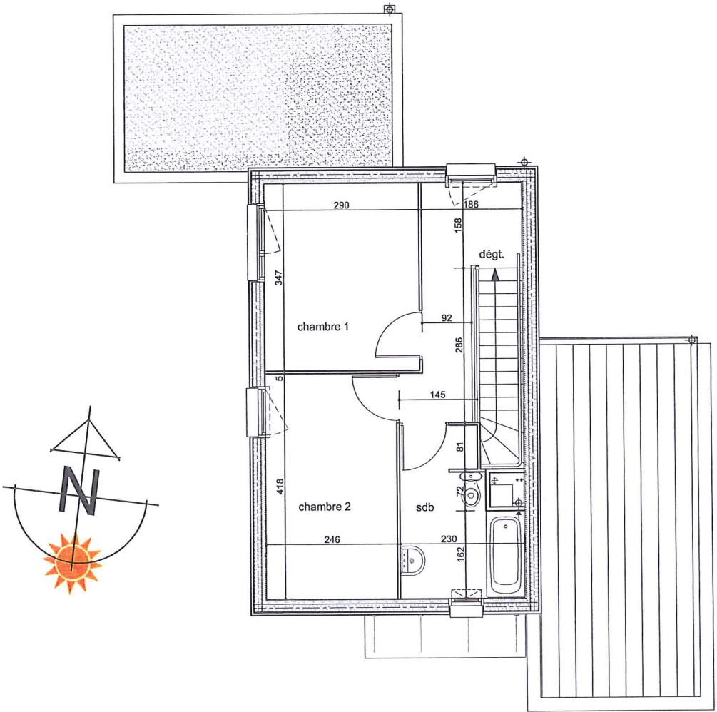
PLAN DE L'ETAGE éch: 1/100
