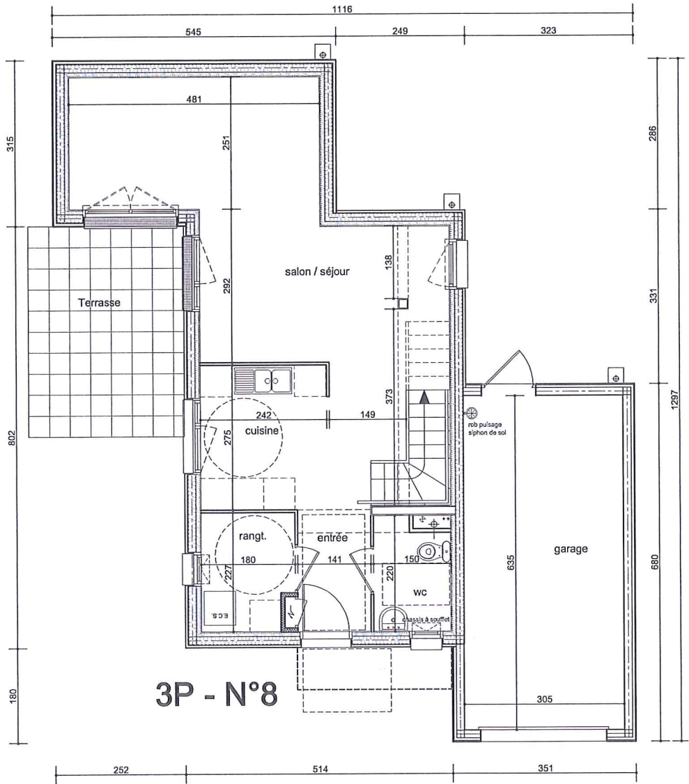
PLAN DU REZ DE CHAUSSEE éch: 1/100
