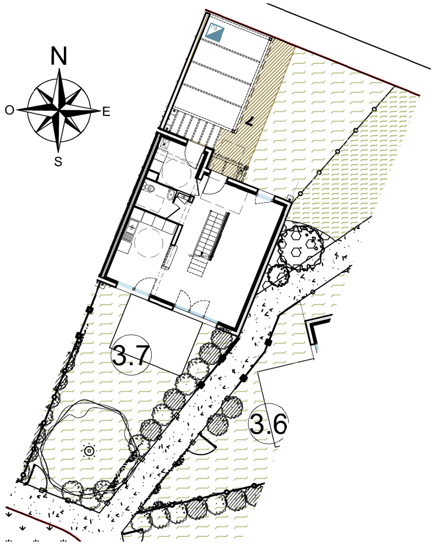
PLAN DE MASSE Superficie de la parcelle : 3.7 : 194m² environ éch : 1/200
