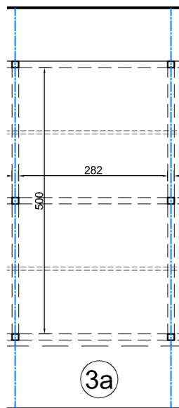
PLAN CARPORT éch : 1/100
