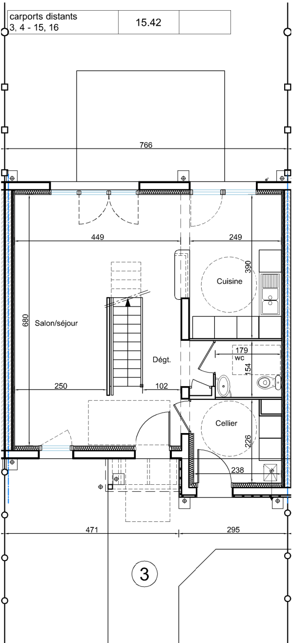
PLAN DU REZ DE CHAUSSEE éch : 1/100
