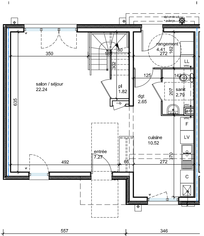
PLAN REZ-DE-CHAUSSEE - éch: 1/100
