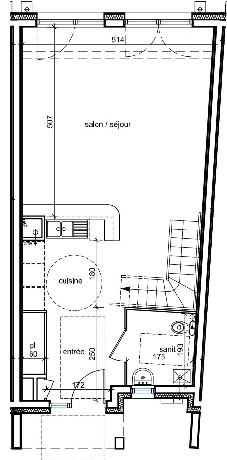
PLAN REZ-DE-CHAUSSEE - éch: 1/100
