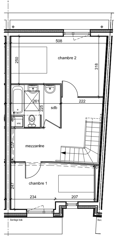
PLAN ETAGE - éch: 1/100
