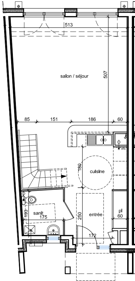
PLAN REZ-DE-CHAUSSEE - éch: 1/100
