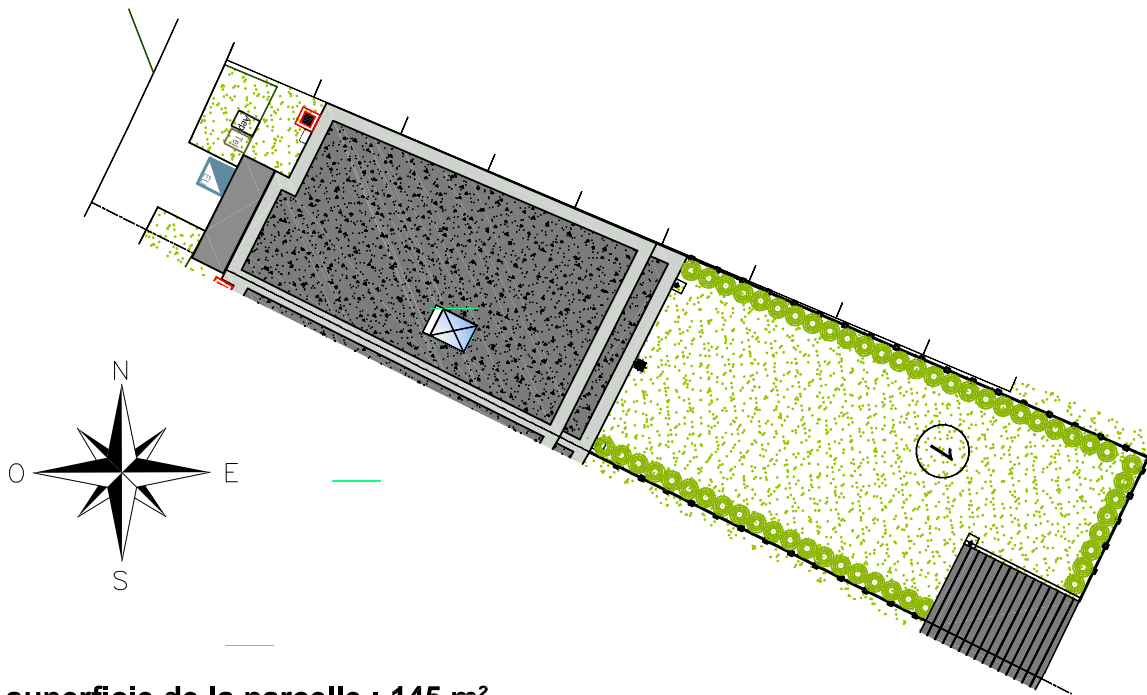
superficie de la parcelle : 145 m² PLAN DE MASSE - éch: 1/200
