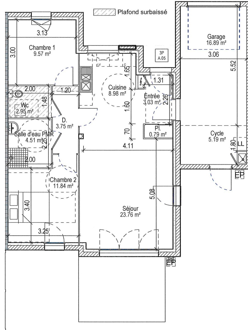
Rez-de-chaussée 1 : 100
