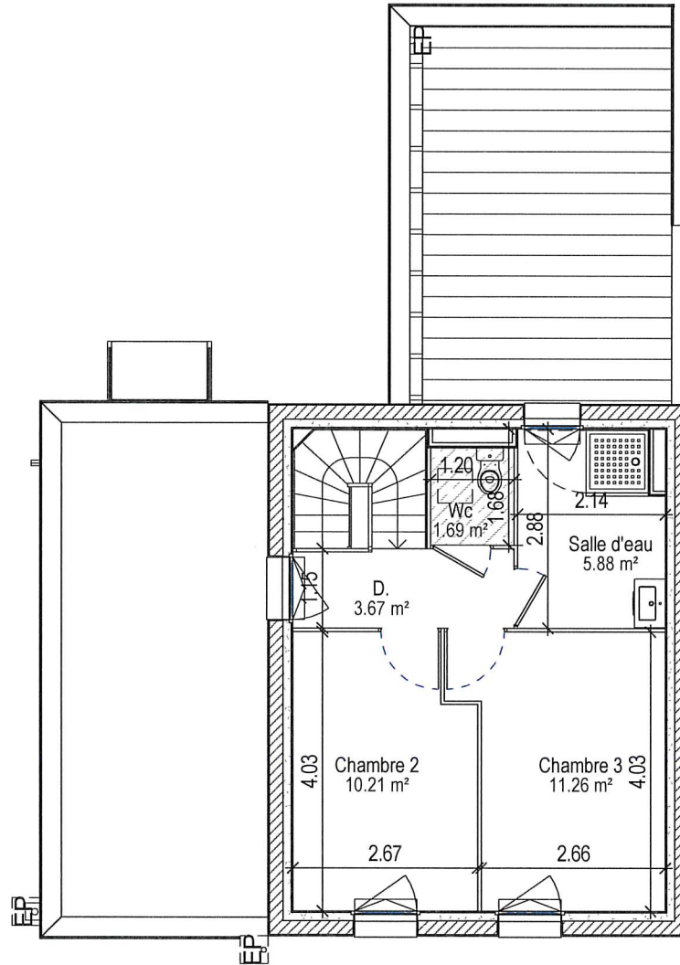
Etage 1 : 100
