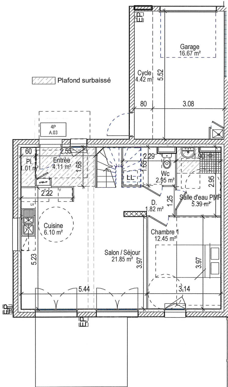
Rez-de-chaussée 1 : 100
