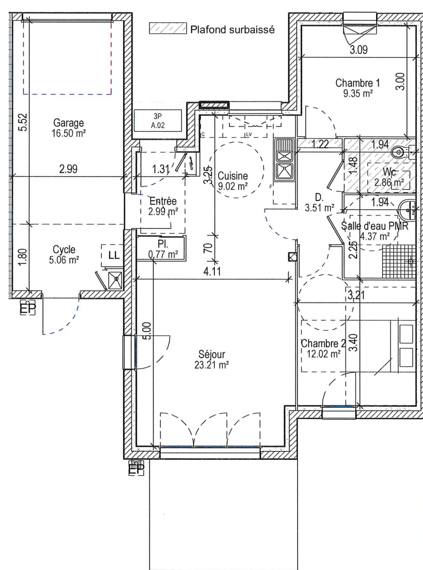
Rez-de-chaussée 1 : 100
