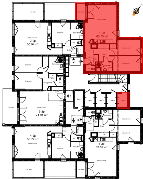
Plan de repérage Etage 1
