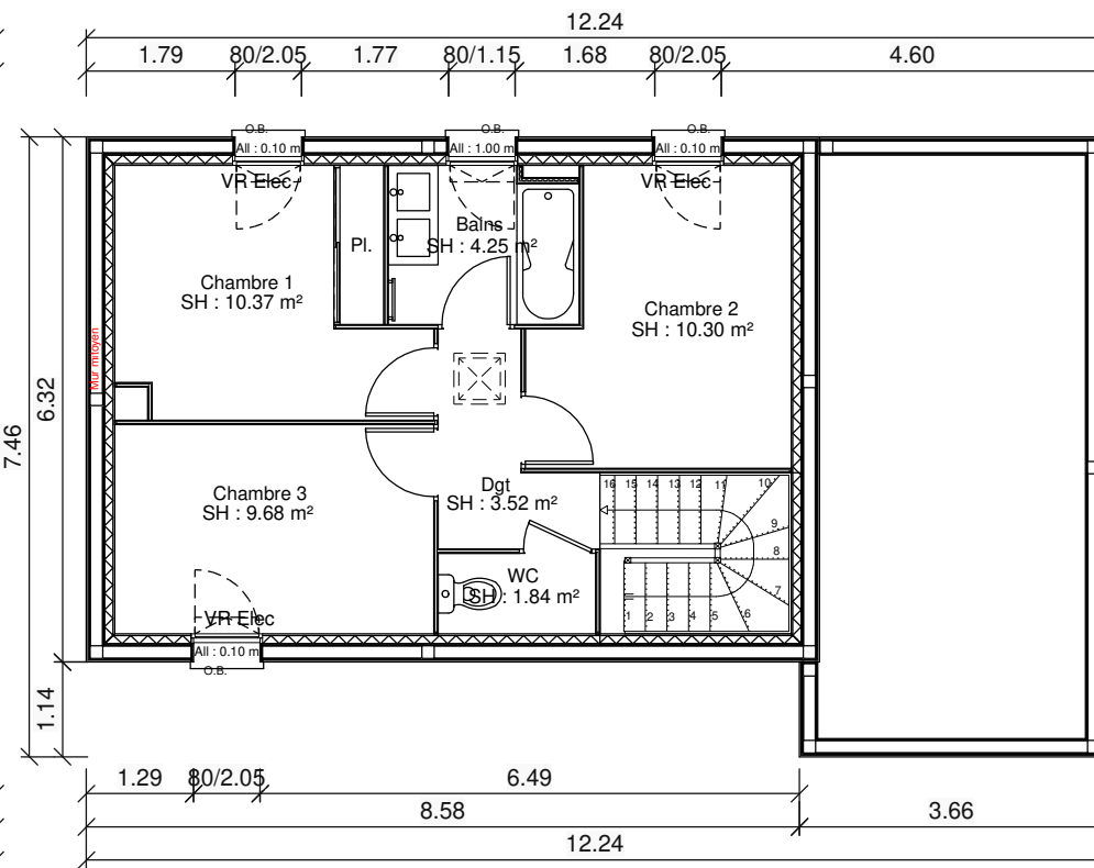
Etage - 1/100
