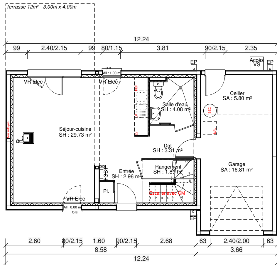
RDC - 1/100
