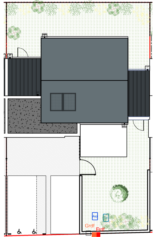
parcelle H4- 246m 2 jardin 92m 2 PLAN DE MASSE 1 2 5
