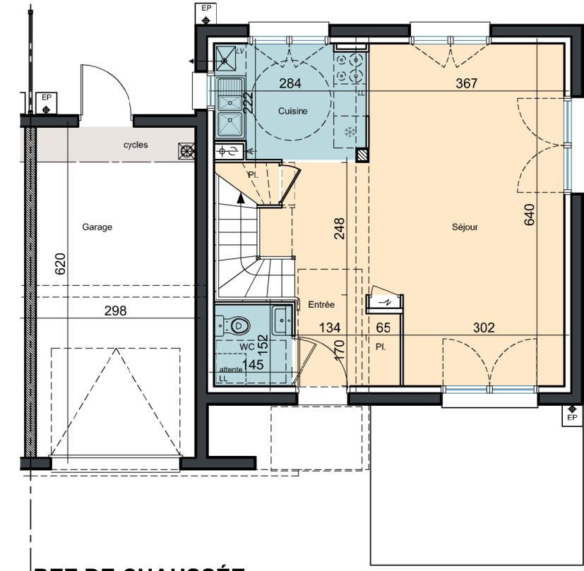
REZ DE CHAUSSÉE
