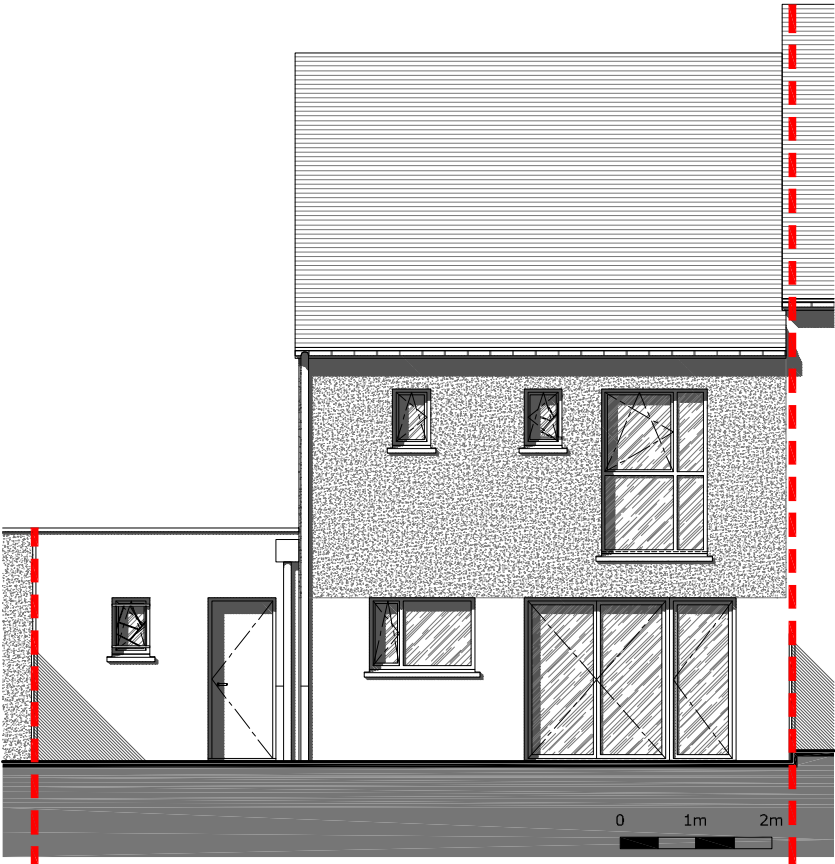
Façade Nord
