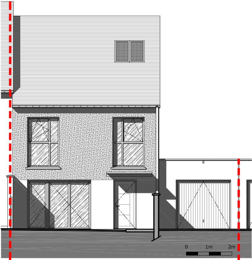
Façade Sud
