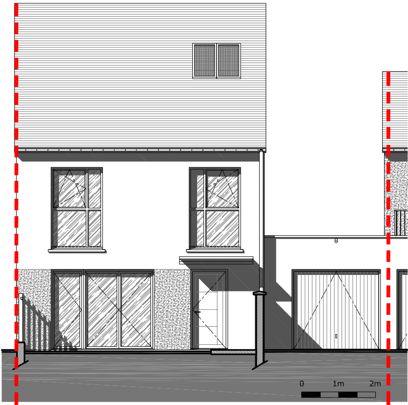
Façade Sud
