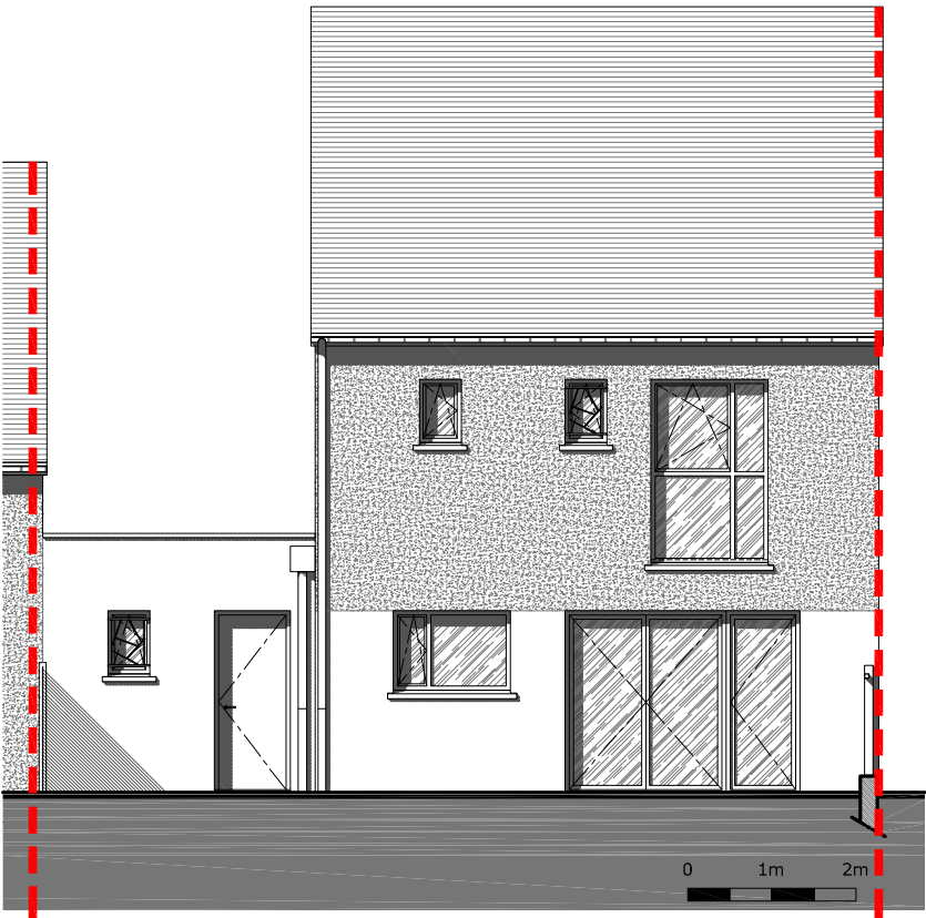
Façade Nord
