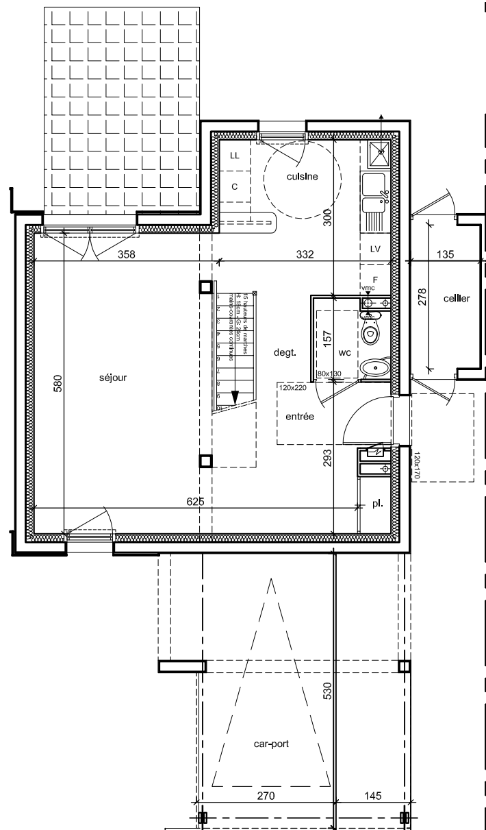
PLAN REZ-DE-CHAUSSEE - éch: 1/100
