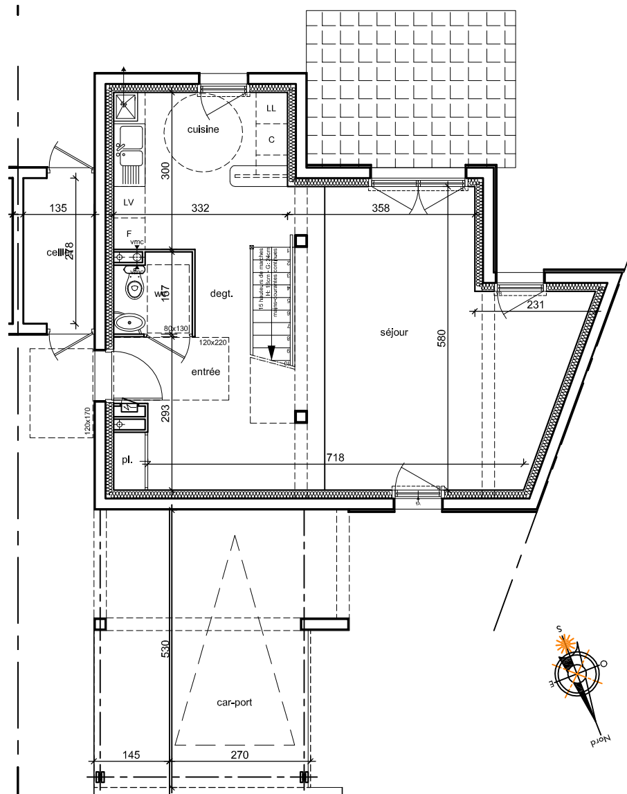
PLAN REZ-DE-CHAUSSEE - éch: 1/100
