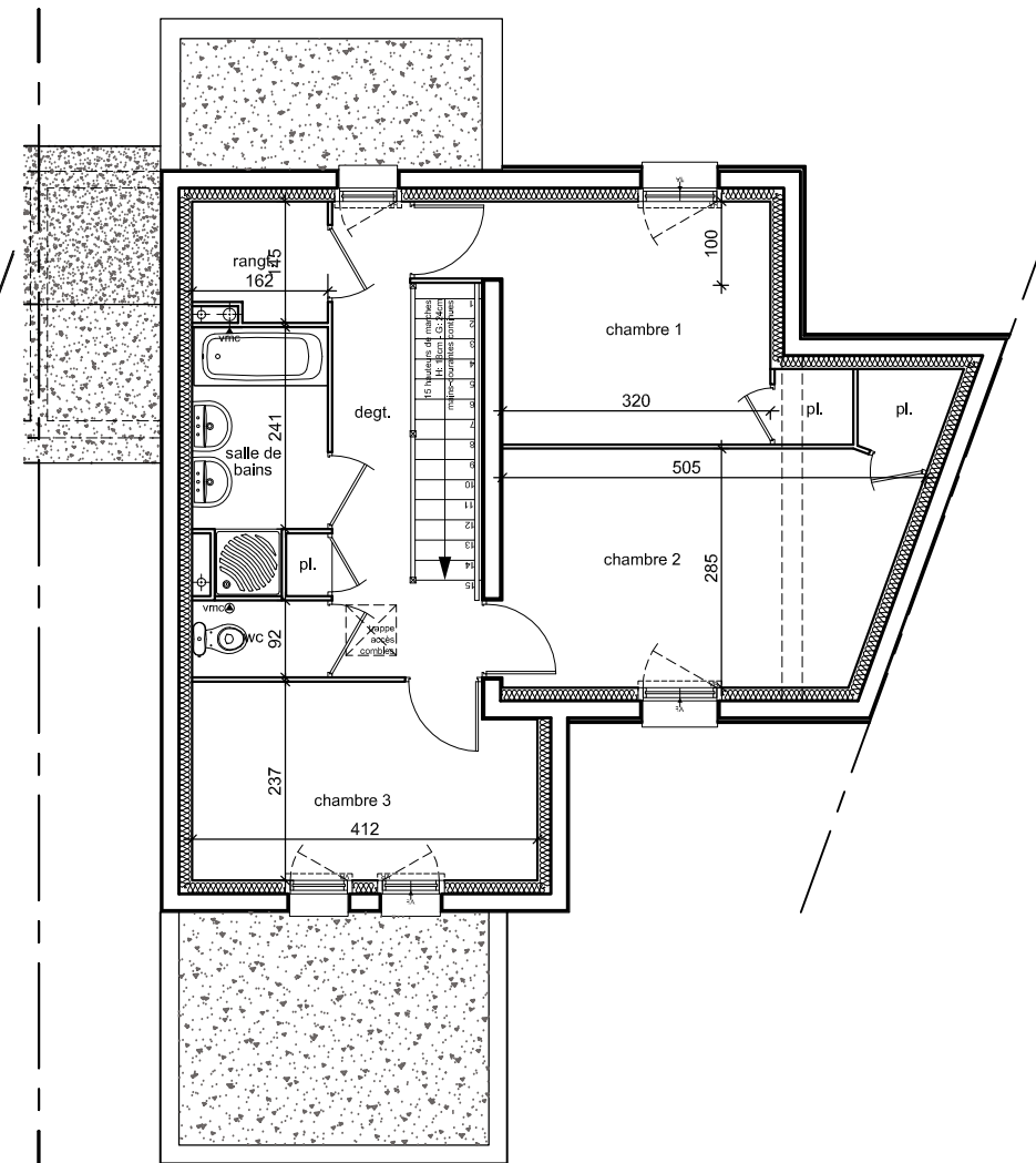
PLAN ETAGE - éch: 1/100
