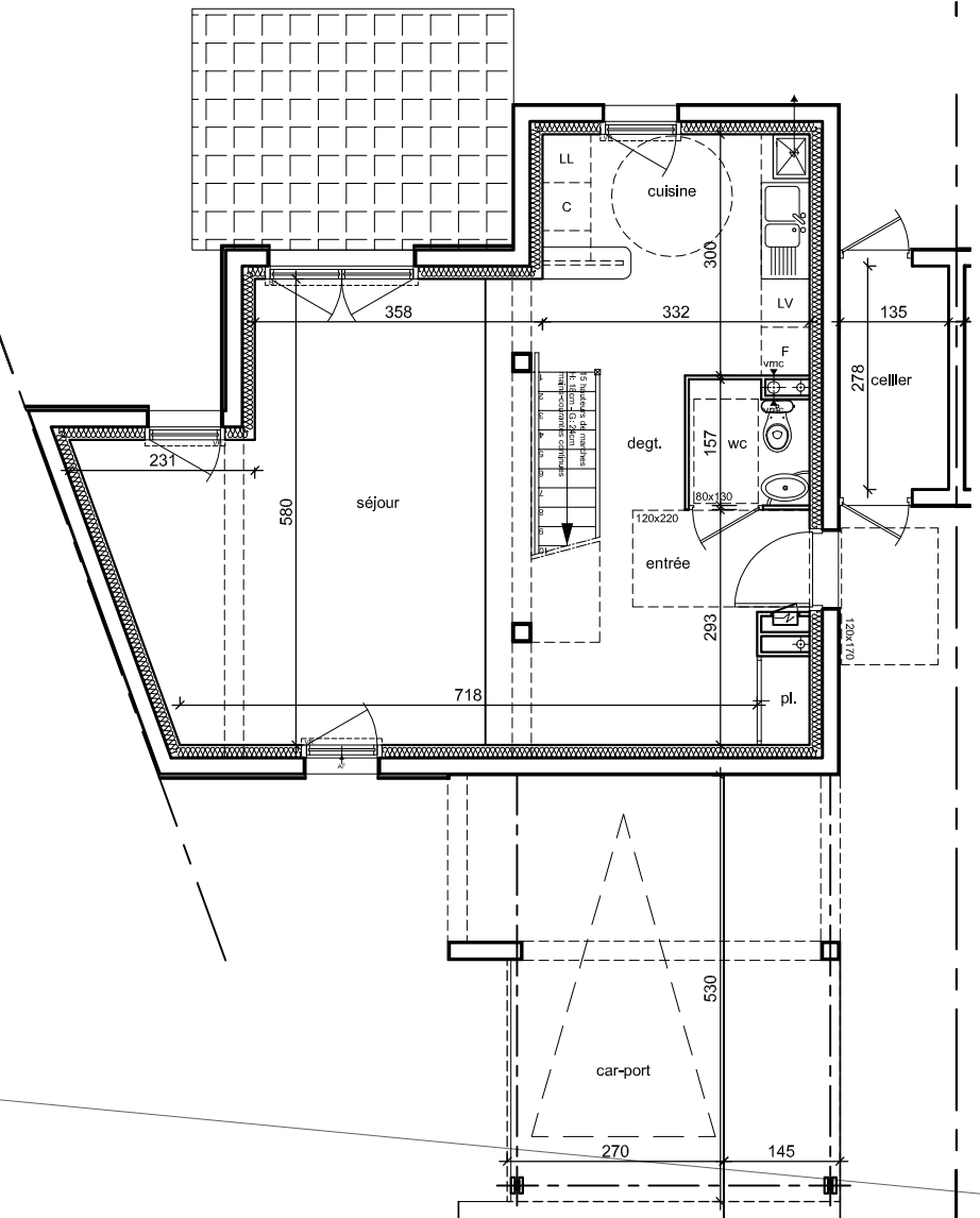
PLAN REZ-DE-CHAUSSEE - éch: 1/100
