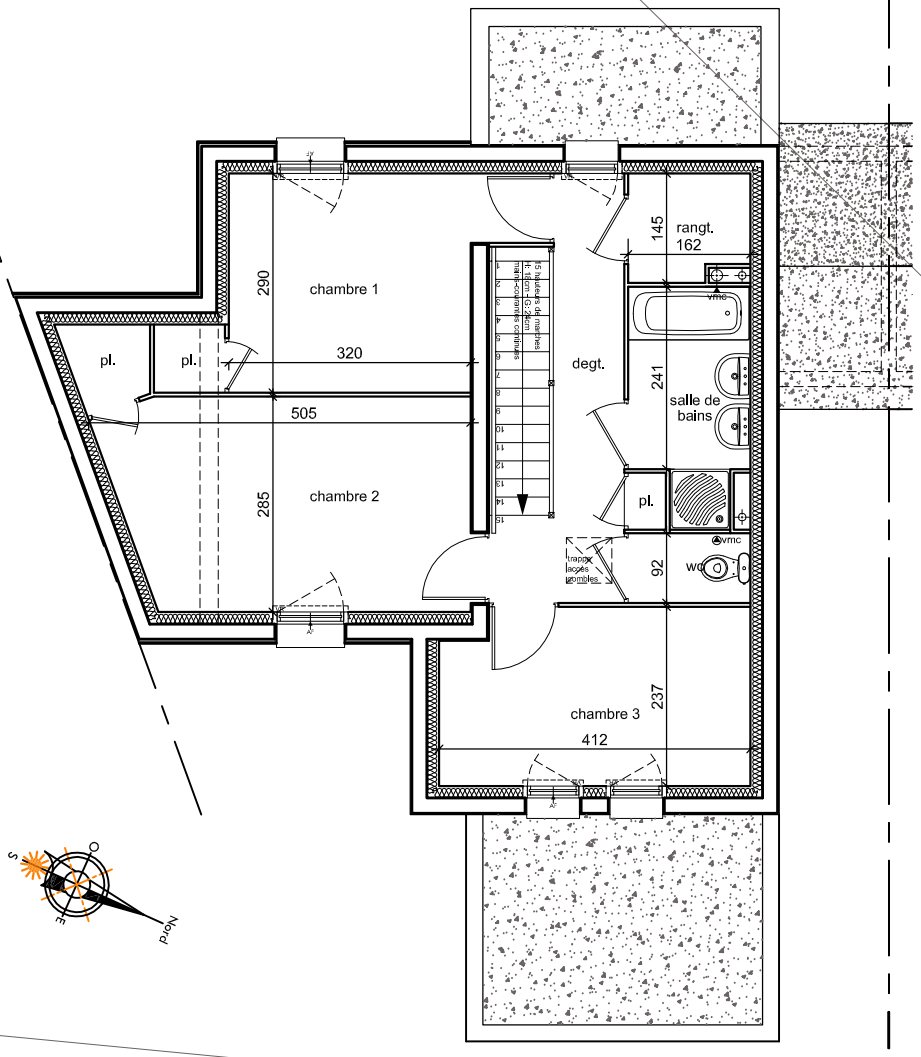
PLAN ETAGE - éch: 1/100
