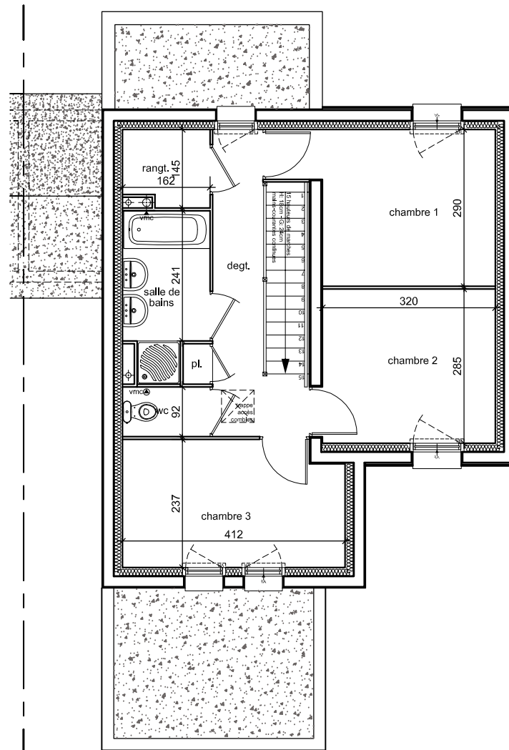
PLAN ETAGE - éch: 1/100
