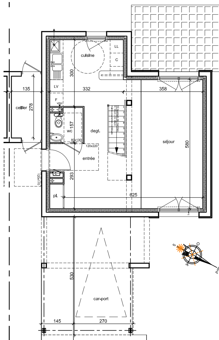
PLAN REZ-DE-CHAUSSEE - éch: 1/100
