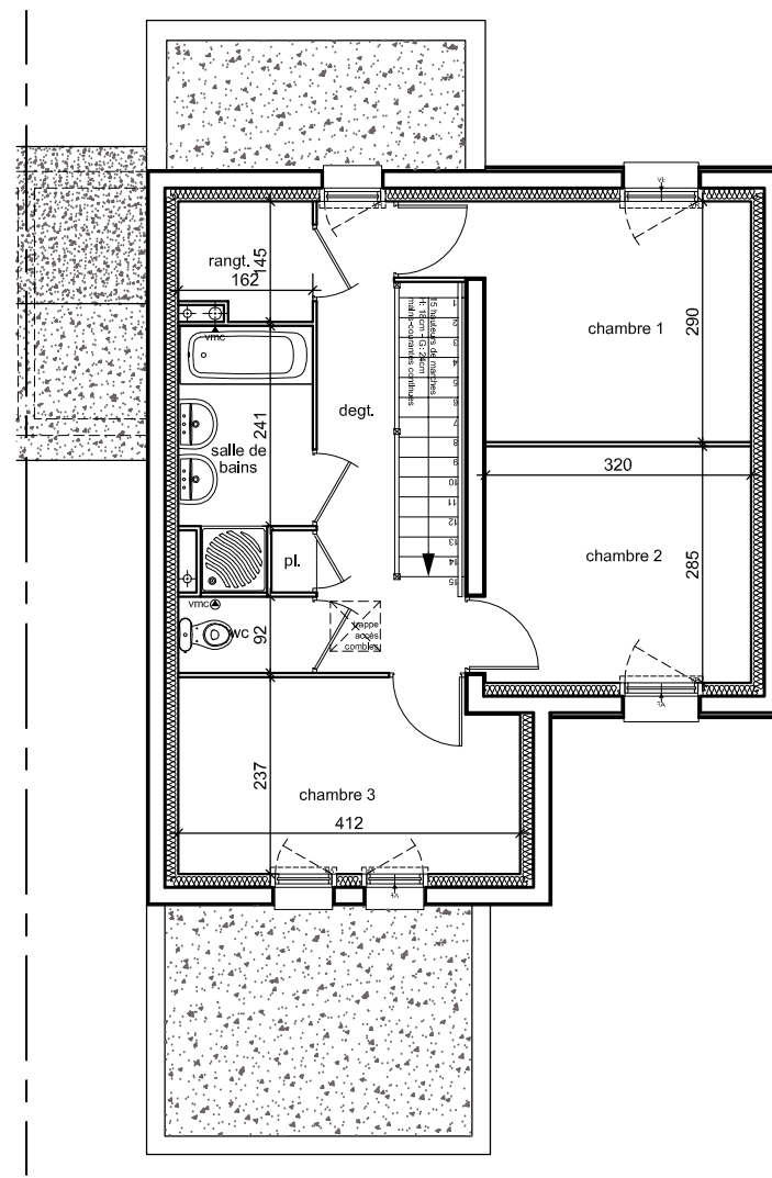
PLAN ETAGE - éch: 1/100
