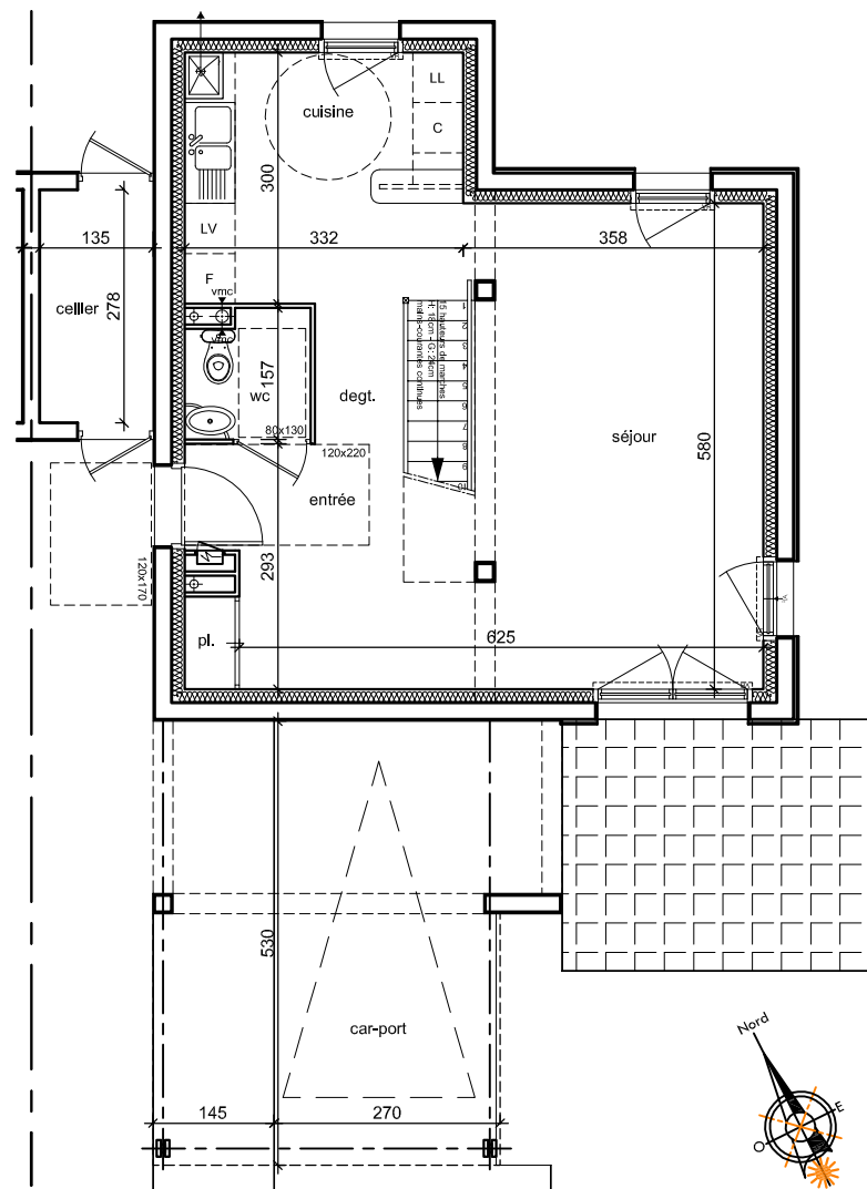
PLAN REZ-DE-CHAUSSEE - éch: 1/100
