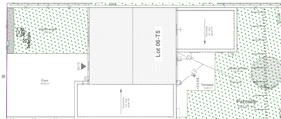
1:200 Plan de masse
