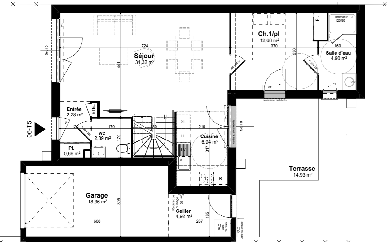
1:100 Rez de chaussée
