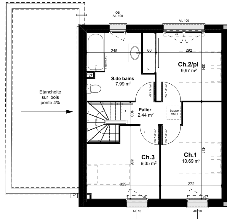
1:100 Etage
