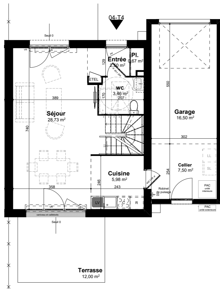
1:100 Rez de chaussée
