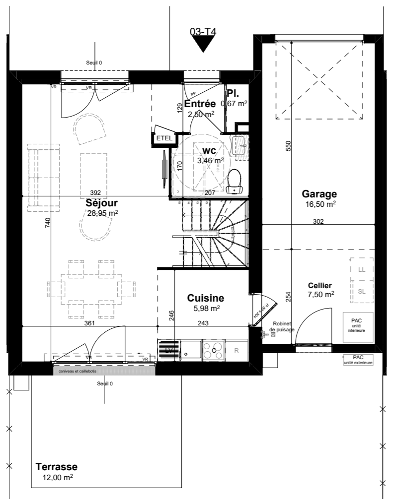
1:100 Rez de chaussée
