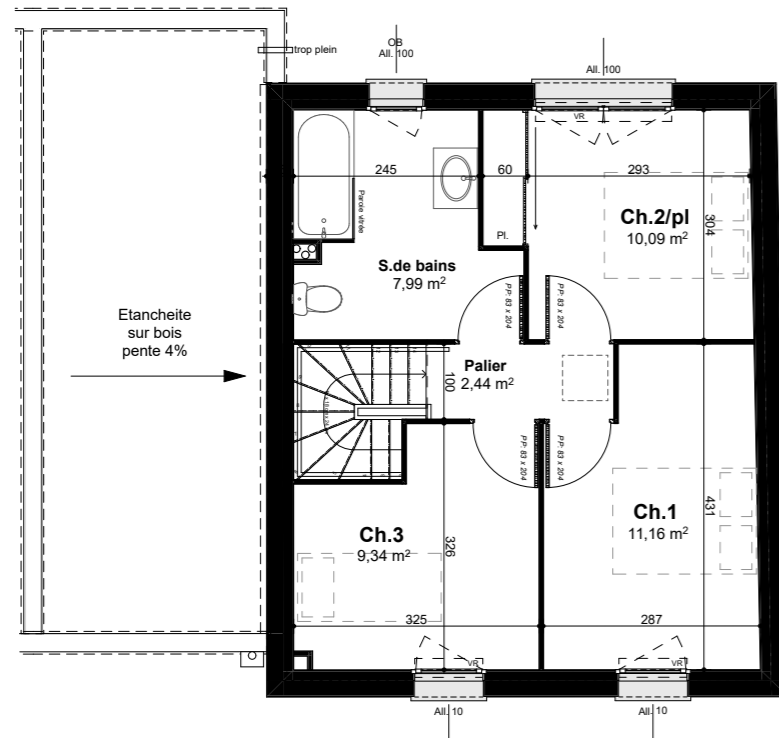
1:100 Etage
