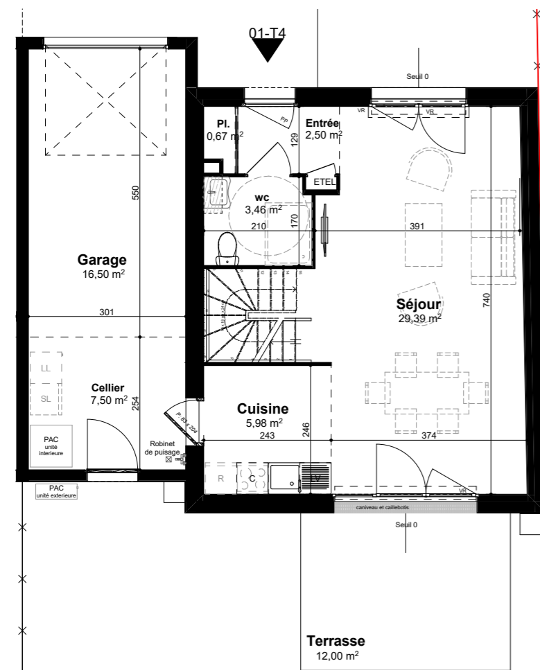
1:100 Rez de chaussée
